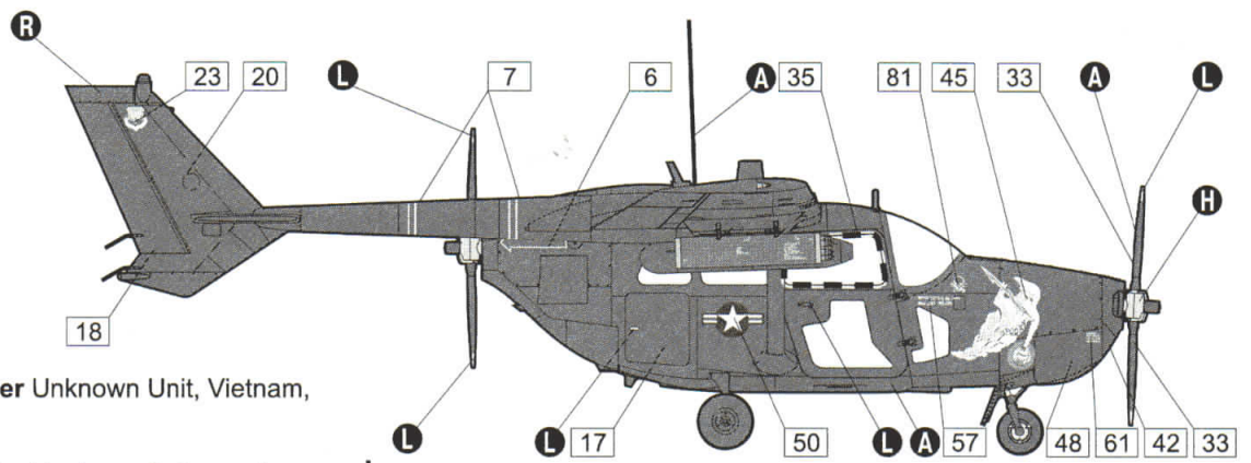
Cessna O-2A Skymaster Невідомий підрозділ, В'єтнам, 1971 рік
