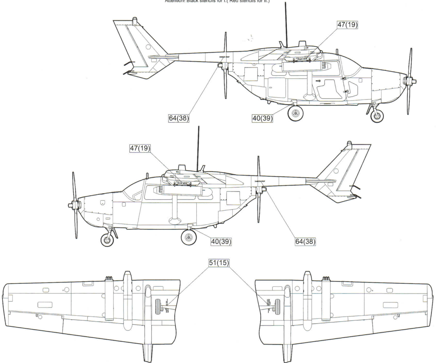
Схема розфарбування і маркування озброєння Scheme of coloring and marking of weapons
